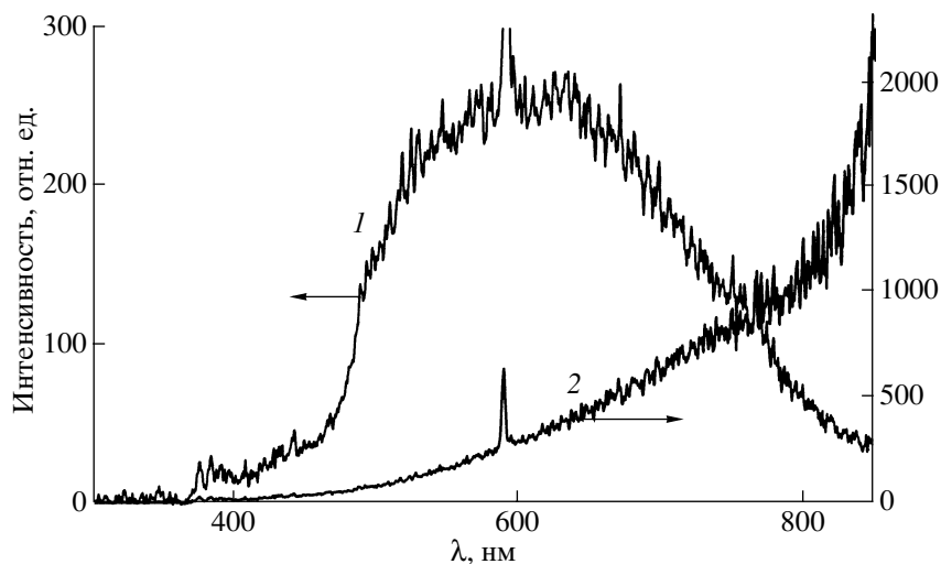
Рис. 2. Спектр излучения СВЧ-разряда в смеси Fe + Al 2 O 3 до ( I ) и после ( 2 ) коррекции.
